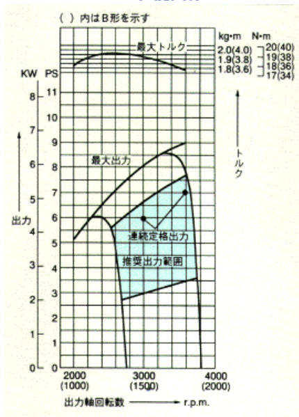
性能曲線
